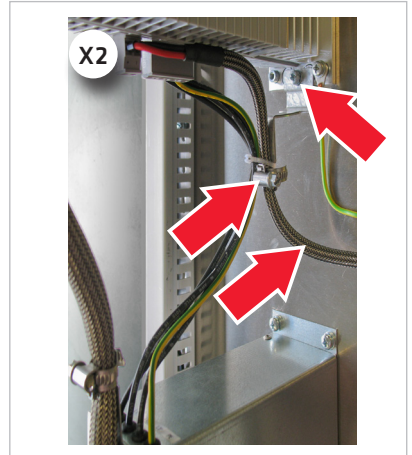
Abbildung 17.2 Musteraufbau - Detail 2: Steuerversorgung
