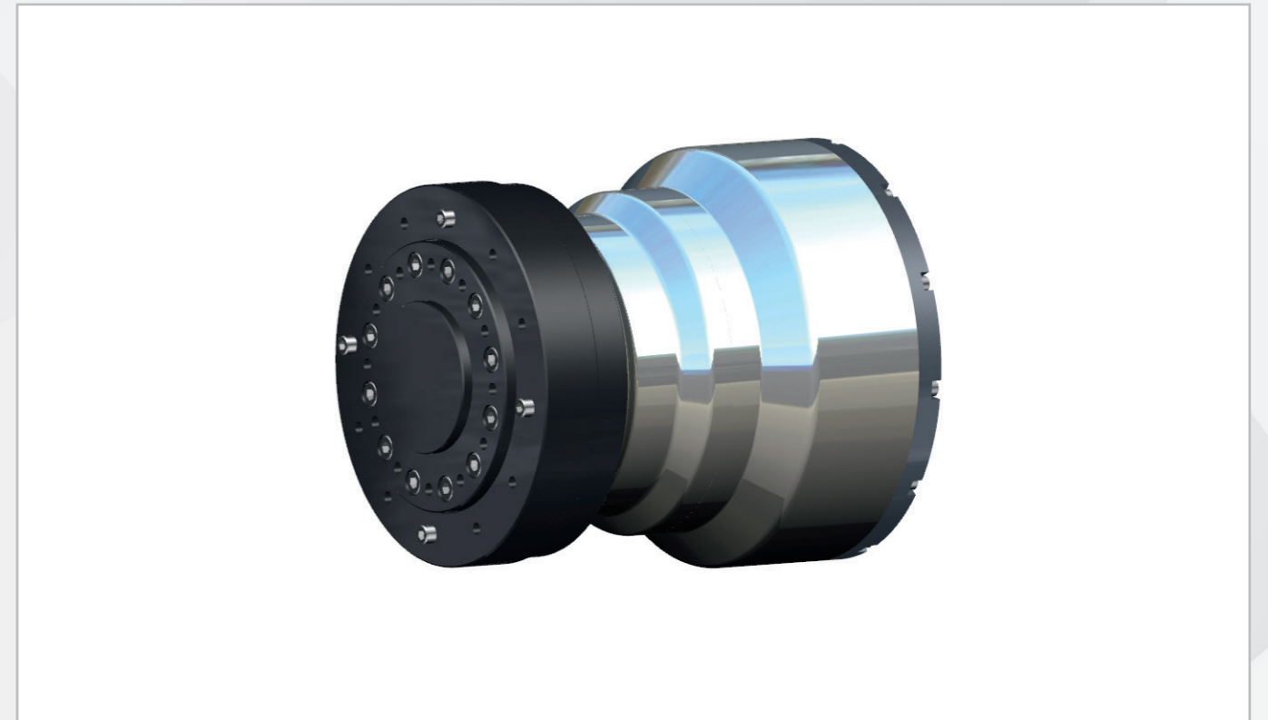
AlopexDrive Aktuator mit integriertem Regler, gesondertem Oberflächenschutz und Materialien für Meerwasserumgebungen
