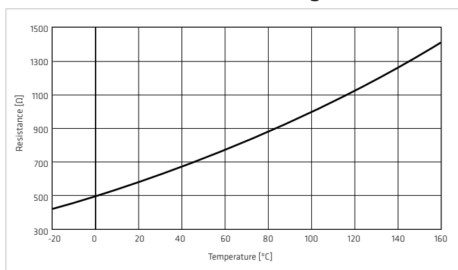
Diagram KTY 84-130
