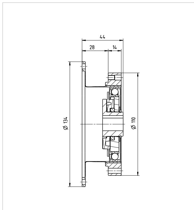
HFUS-32-2A [mm]
