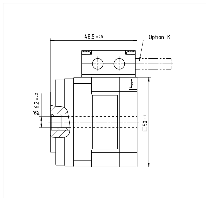
FHA-8C Mini [mm]
