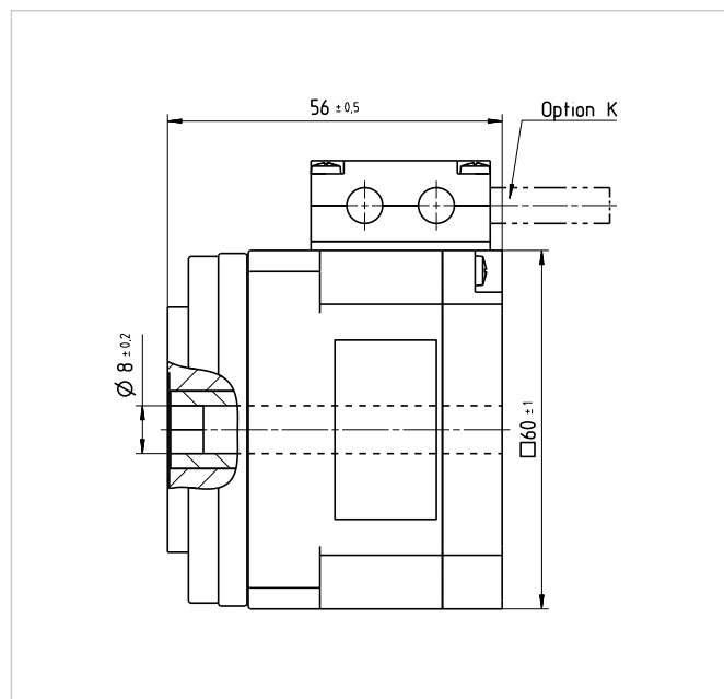
FHA-11C Mini [mm]
